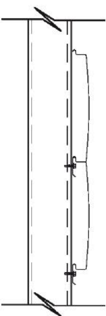
PANEL D 20 200 ARQUITECTÓNICO REVESTIMIENTO HORIZONTAL - VERTICAL
