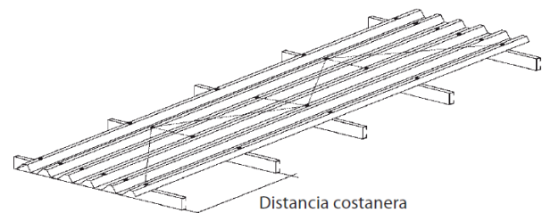
FIJACION GANCHO OMEGA
