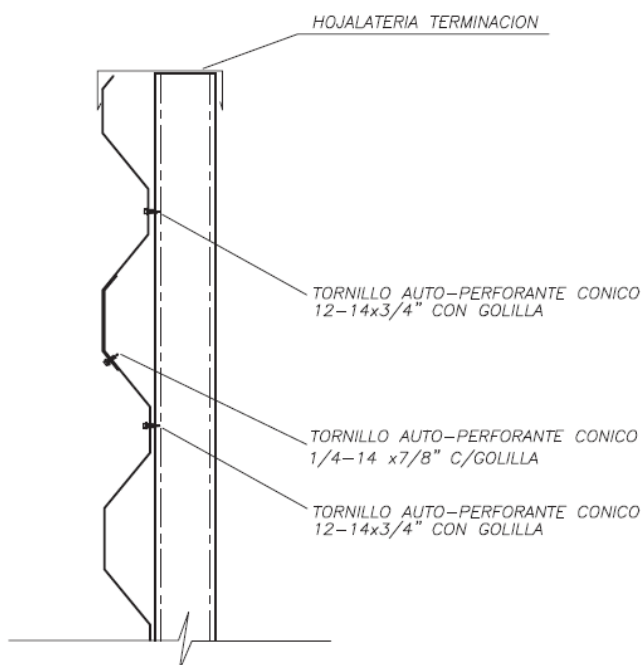
DETALLE FIJACION REVESTIMIENTO HORIZONTAL
