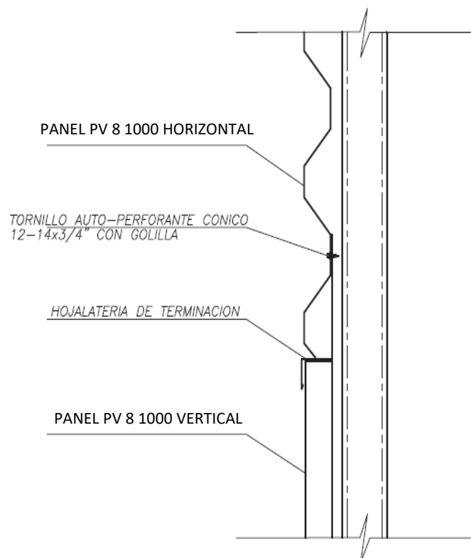
DETALLE REVESTIMIENTO HORIZONTAL Y VERTICAL
